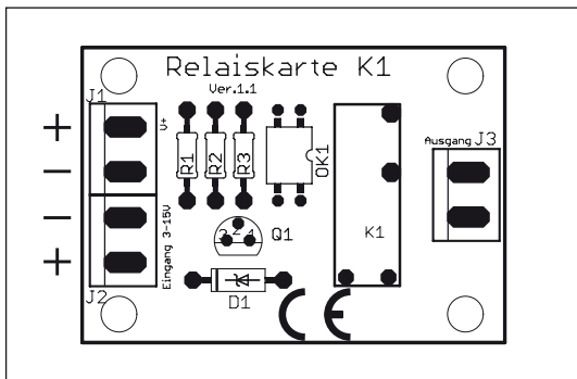
Platinenlayout für die Relaiskarte K1
