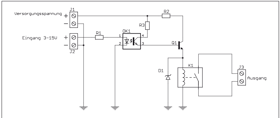
Schaltplan für die Relaiskarte K1
